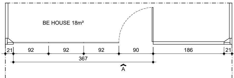
PLANTA VIDRAÇARIA - BE HOUSE 18m² ESCALA 1/50
