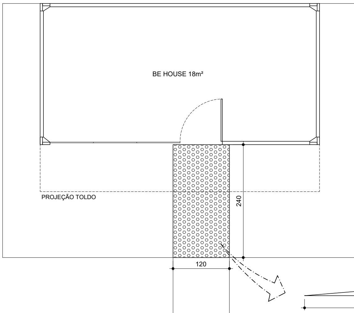
PLANTA ACESSIBILIDADE - BE HOUSE 18m² ESCALA 1/50
