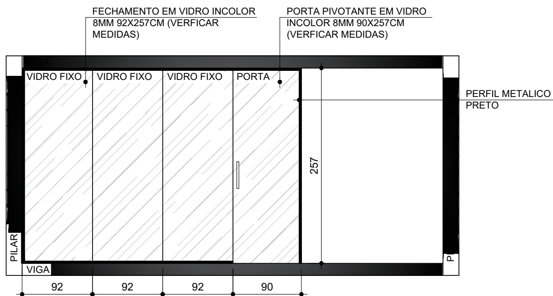
VISTA A ESCALA 1/50
