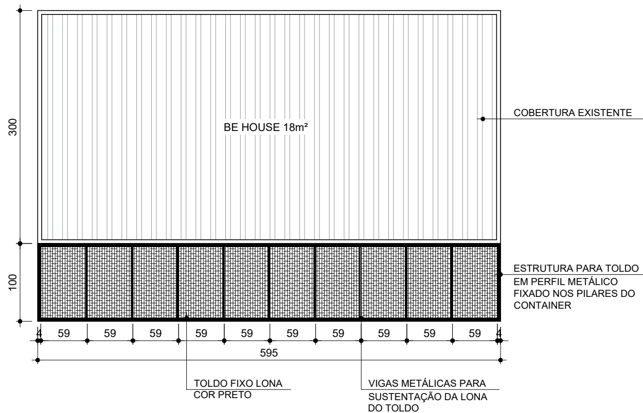
PLANTA COBERTURA - BE HOUSE 18m² ESCALA 1/50
