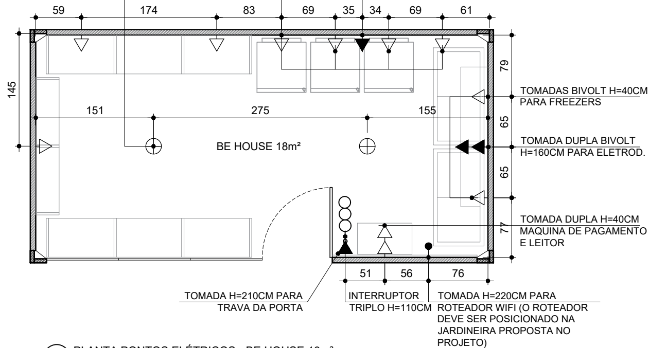
PLANTA PONTOS ELÉTRICOS - BE HOUSE 18m² ESCALA 1/50
