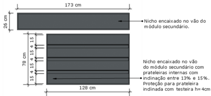
VISTA FRONTAL - NICHOS
