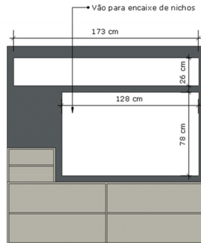
VISTA FRONTAL - NICHOS
