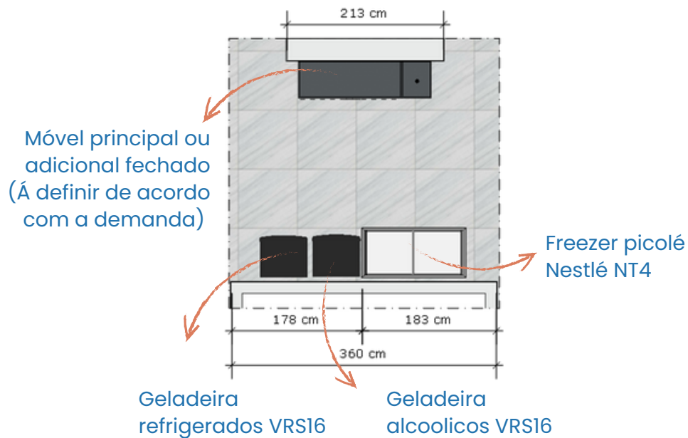
Planta Layout
