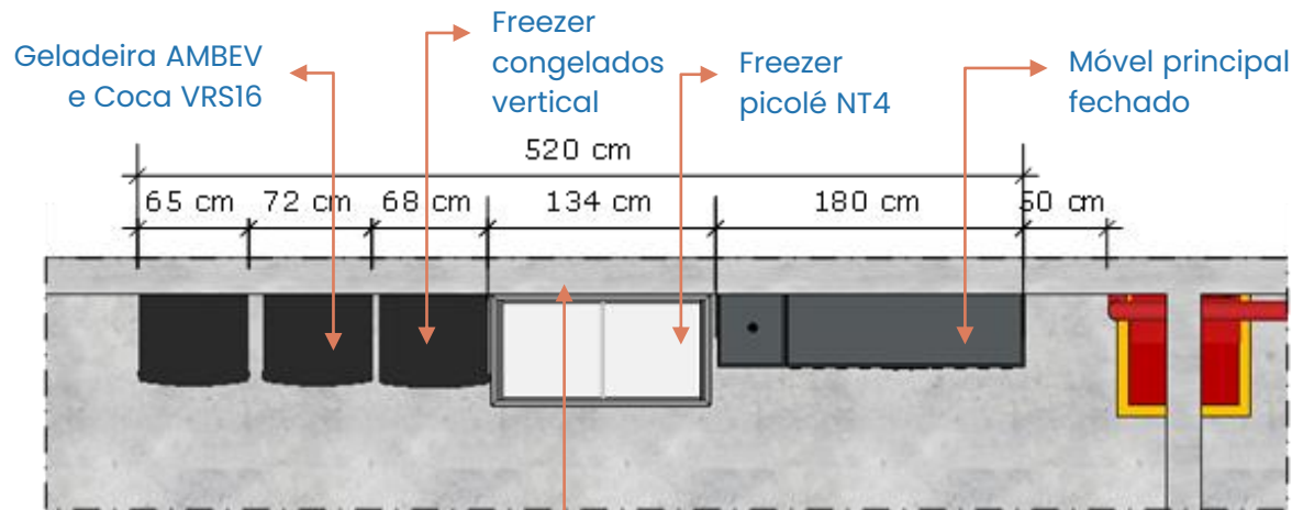
Planta Layout
