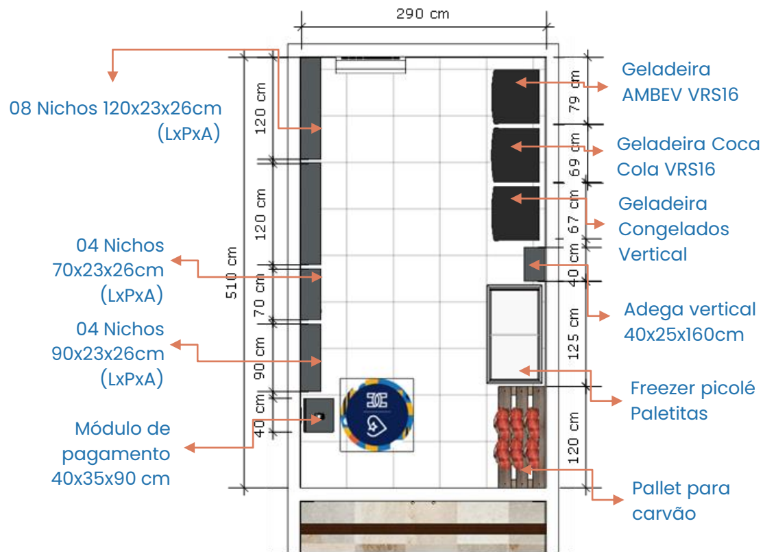
Planta Layout
